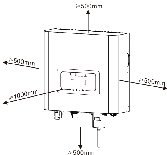
Img4.3 Vãos mínimos para instalação
