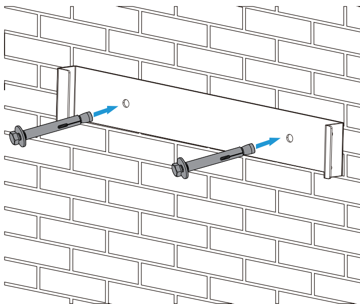
Img4.5 Instalação do braço de montagem
