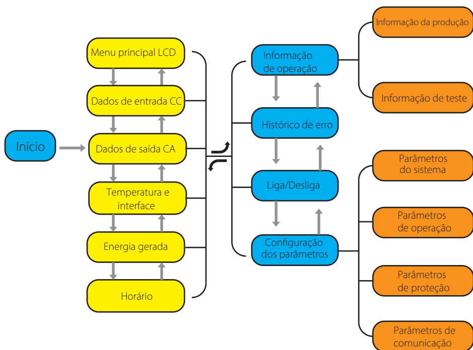
Img8.1 diagrama de operação do display LCD
