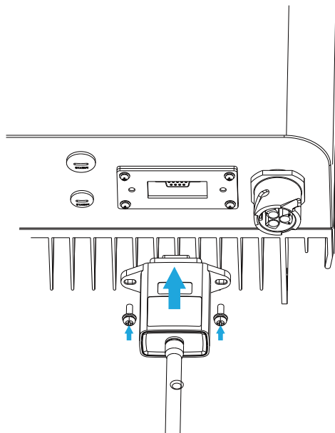
Img5.13 Instalação do plugue Wi-Fi
