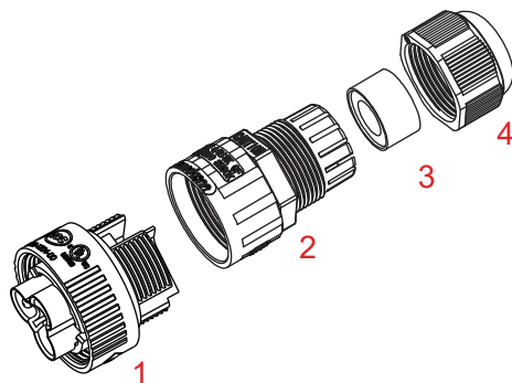
Img5.7 Estrutura do conector CA
