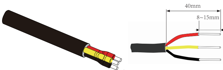
Img5.8 Cabo CA decapado
