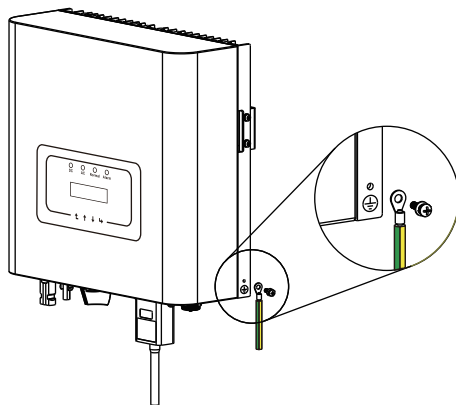
Img5.11 Aterramento da carcaça do inversor
