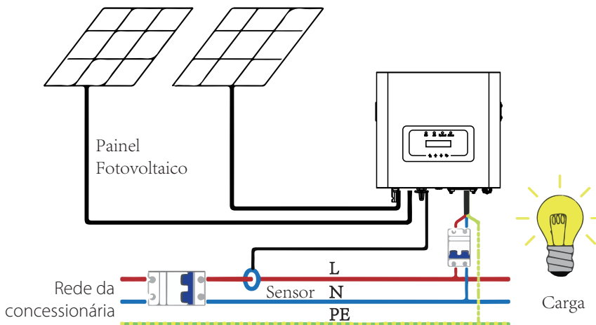
Img7.1 Diagrama de conexão do Limiter
