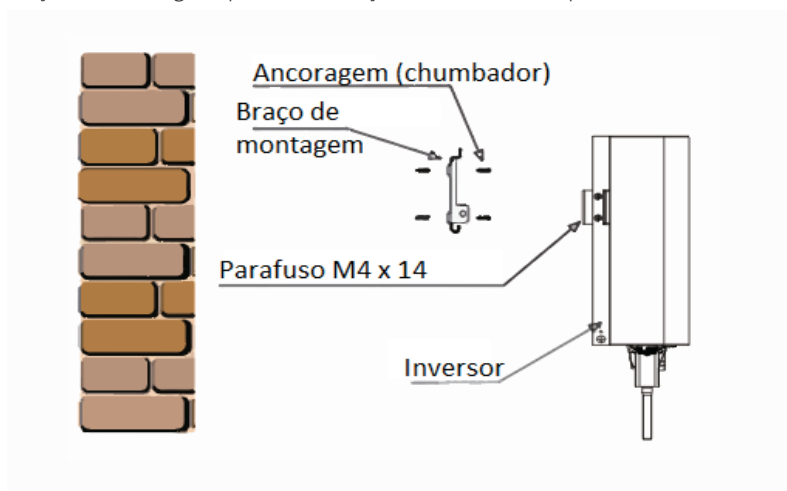
Img4.4 Instalação do inversor
