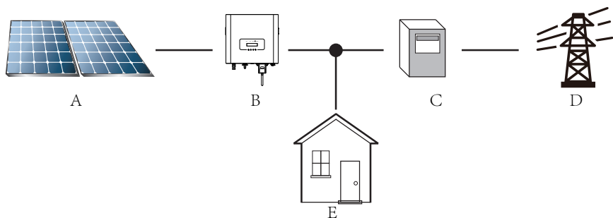
Exemplo da aplicação de inversor fotovoltaico em sistema
