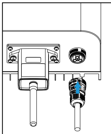
Img5.10 Conexão CA com o inversor
