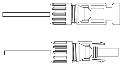
Img5.5 Conector CC com a rosca afixada
