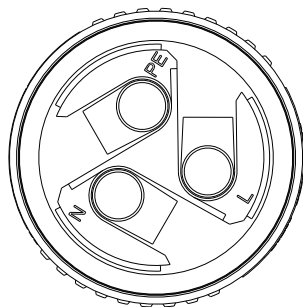
Img5.9 Padrão das conexões do terminal CA.
